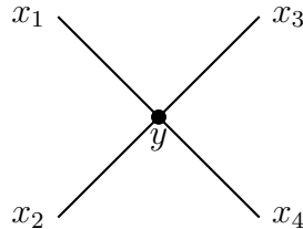
Figura 21.1: Diagramma a un vertice (ordine g ) per la funzione a 4 punti.
